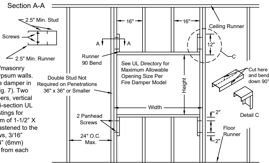
Fig. 3: Metal or Wood Stud Wall
