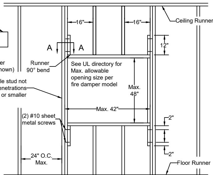
Fig. 2: Metal or Wood Stud Wall
