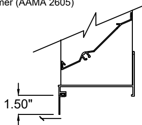
OPTIONAL FLANGE
