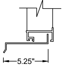
OPTIONAL EXTENDED SILL
